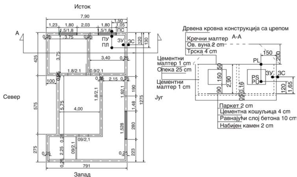
Слика 3. Распоред мерних уређаја типичне сеоске војвођанске куће
