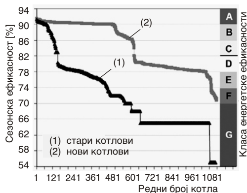
Слика 2. Приказ SEDBUK за преко 2000 котлова
